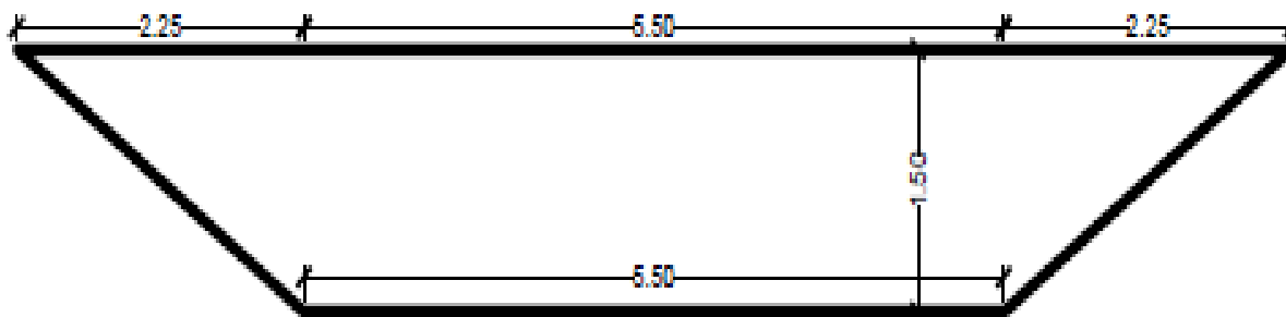
CORTE A-A' RESERVORIO ESC. 1:50
