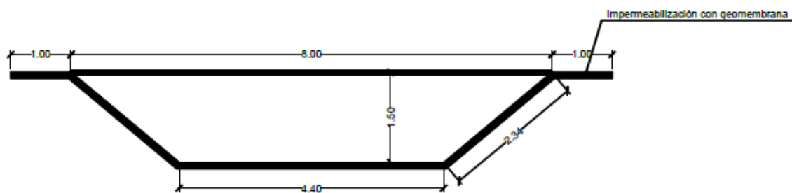
CORTE A-A' RESERVORIO ESC. 1:100
