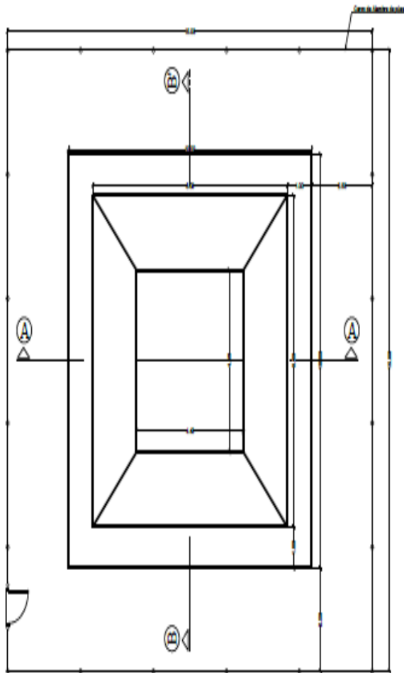
PLANTA RESERVORIO ESC. 1:100
