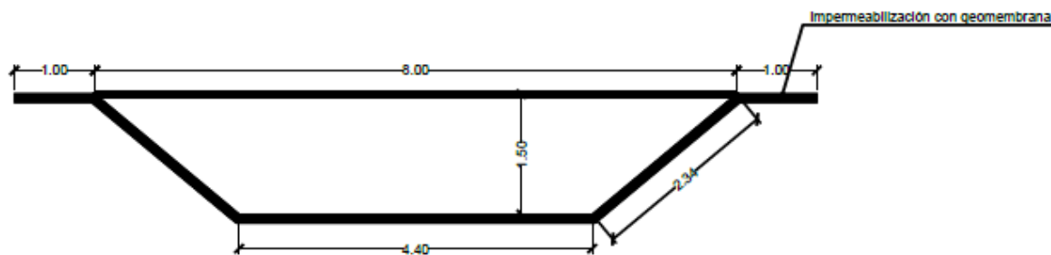
CORTE B-B' RESERVORIO ESC. 1:100
